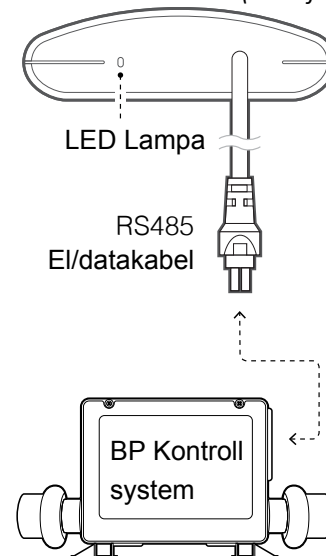
GATEWAY ULTRA Enhet (visas från sidan)
